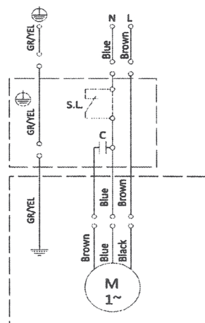
Fig. 8: Diagrammes de raccordement à 3 fils avec cabinet condensateur ( S.L: possible flotteur)
