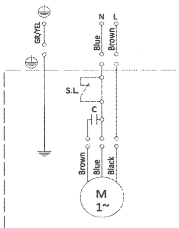
Fig. 7: Diagrammes à 3 fils avec condensateur dans la pompe (seulement VS 40) ( S.L: possible flotteur)
