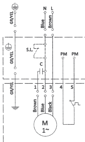
Fig. 9: Diagrammes à 3 fils avec cabinet condensateur avec disjoncteur ( S.L: possible flotteur)
