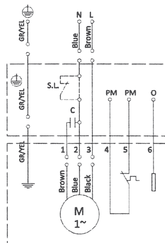
Fig. 10: Diagrammes à 3 fils avec cabinet condensateur avec disjoncteur et le capteur d'huile ( S.L: flotteur)
